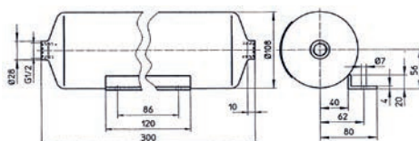
Masszeichnung K 3043
