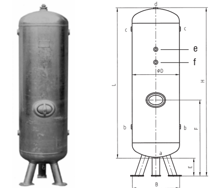
Masszeichnung K 3043
